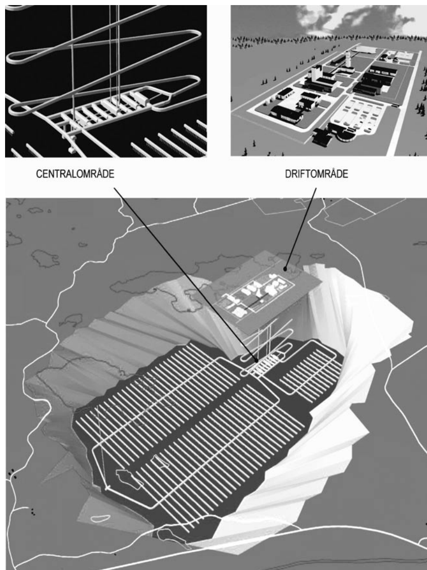
Figur 3-8. Djupförvaret – översikt.
